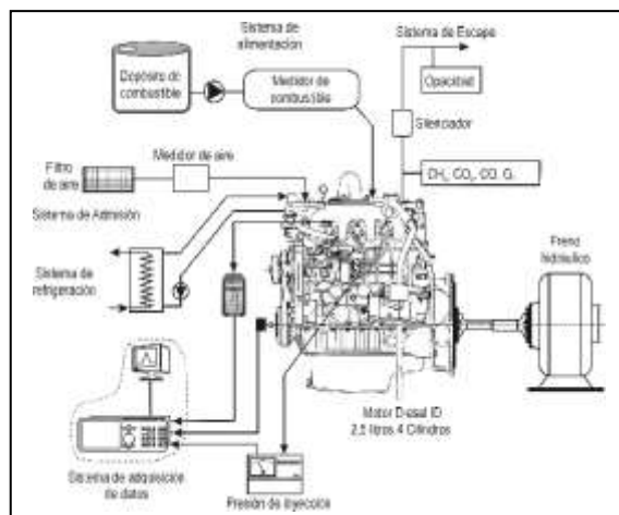
Figura 1. Uso del biodiesel en motores de diésel [2] NORMA ISO Figura 1. Uso del biodiesel en motores de diésel (Sandoval, 2015) NORMA APA
